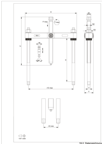
18-3_Datenzeichnung
